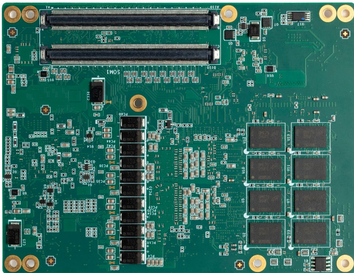
图 1-2 COMe-BSKL-H01 产品图片
