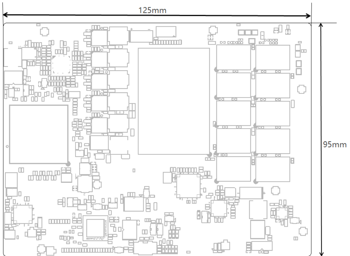
图 5-1 结构尺寸图
