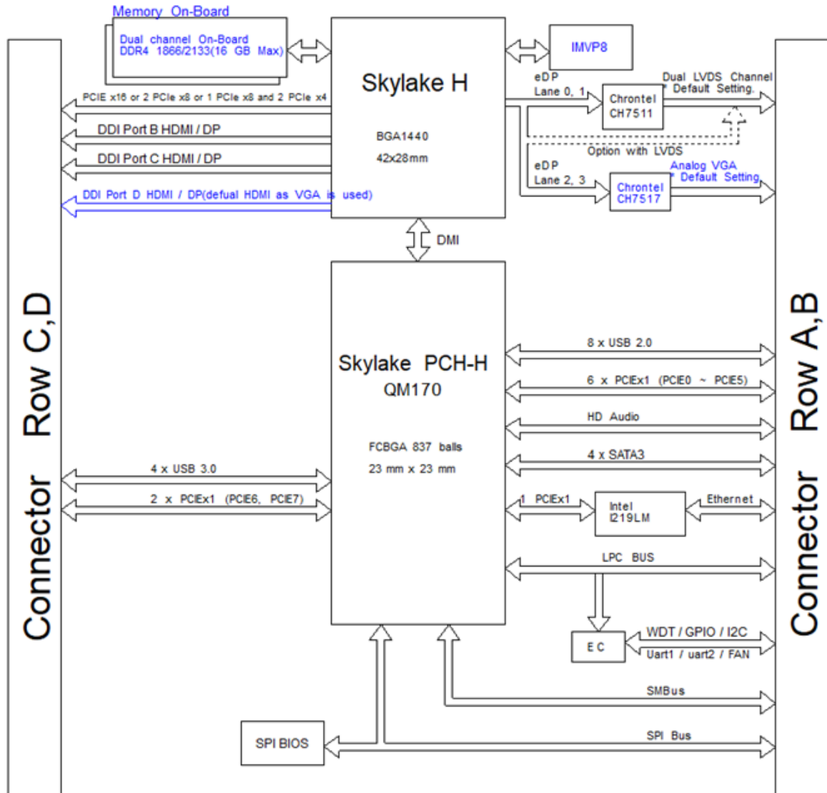
图 1-1 功能模块示意图
