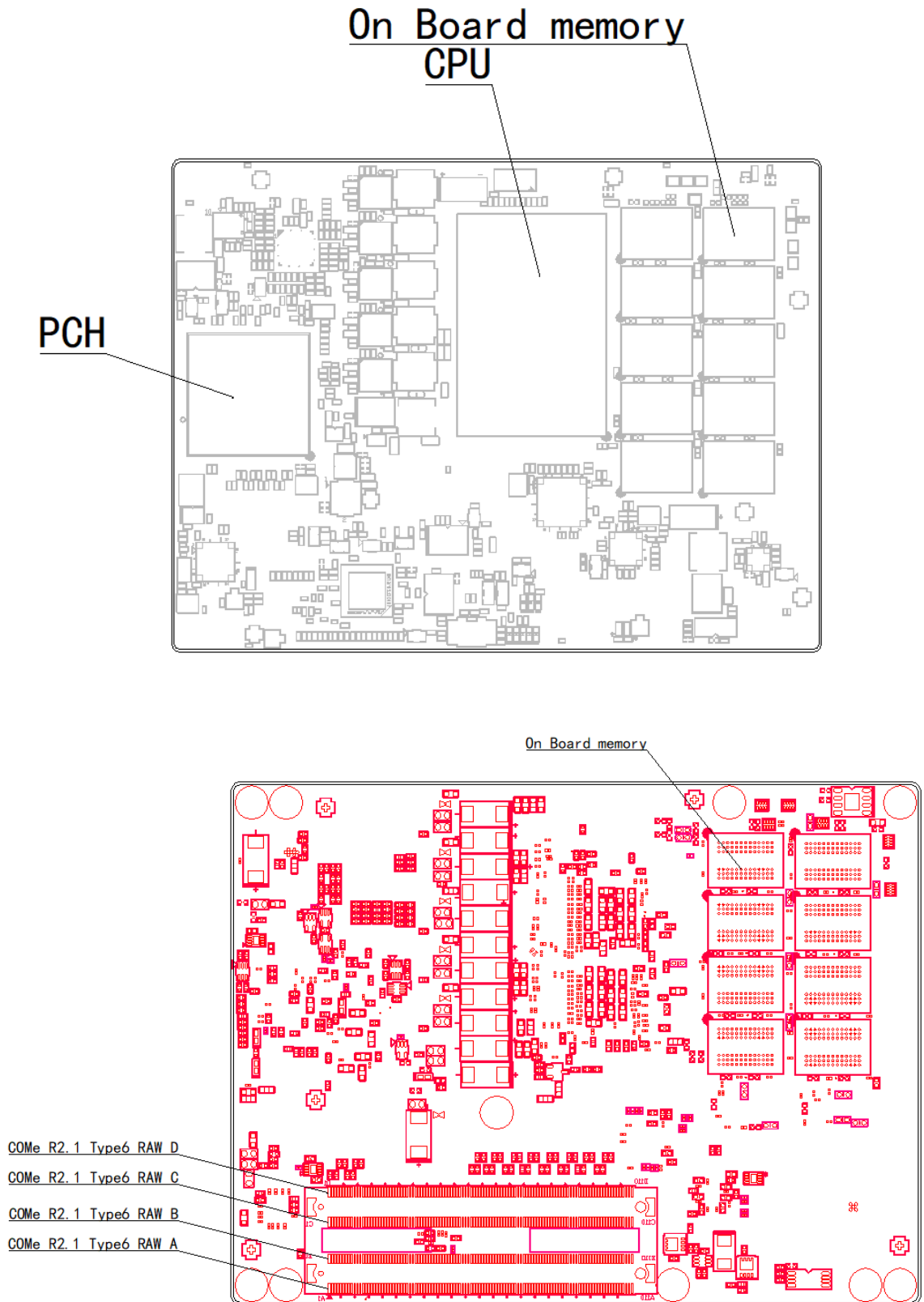
图 3-1 主板正反面接口图
